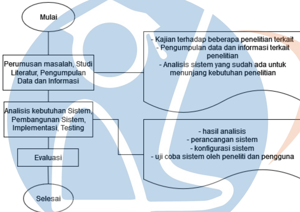
Gambar 3.1 Tahapan Penelitian
