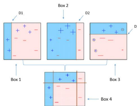
Gambar 2.12 Proses Boosting Dengan Adaboost
