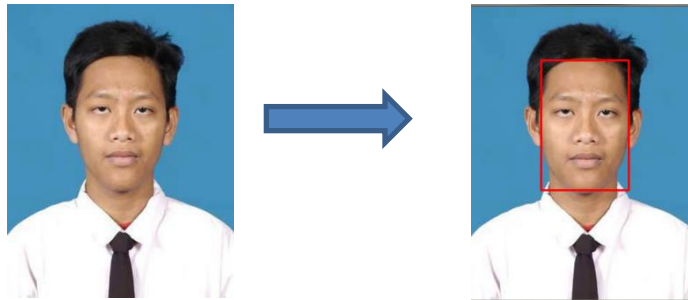
Gambar 2.7 Deteksi Wajah
